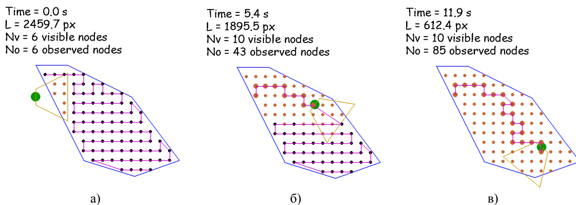
Рис. 3. Этапы построения уточненного маршрута H в процессе имитационного моделирования при втором способе начального расположения БПЛА
